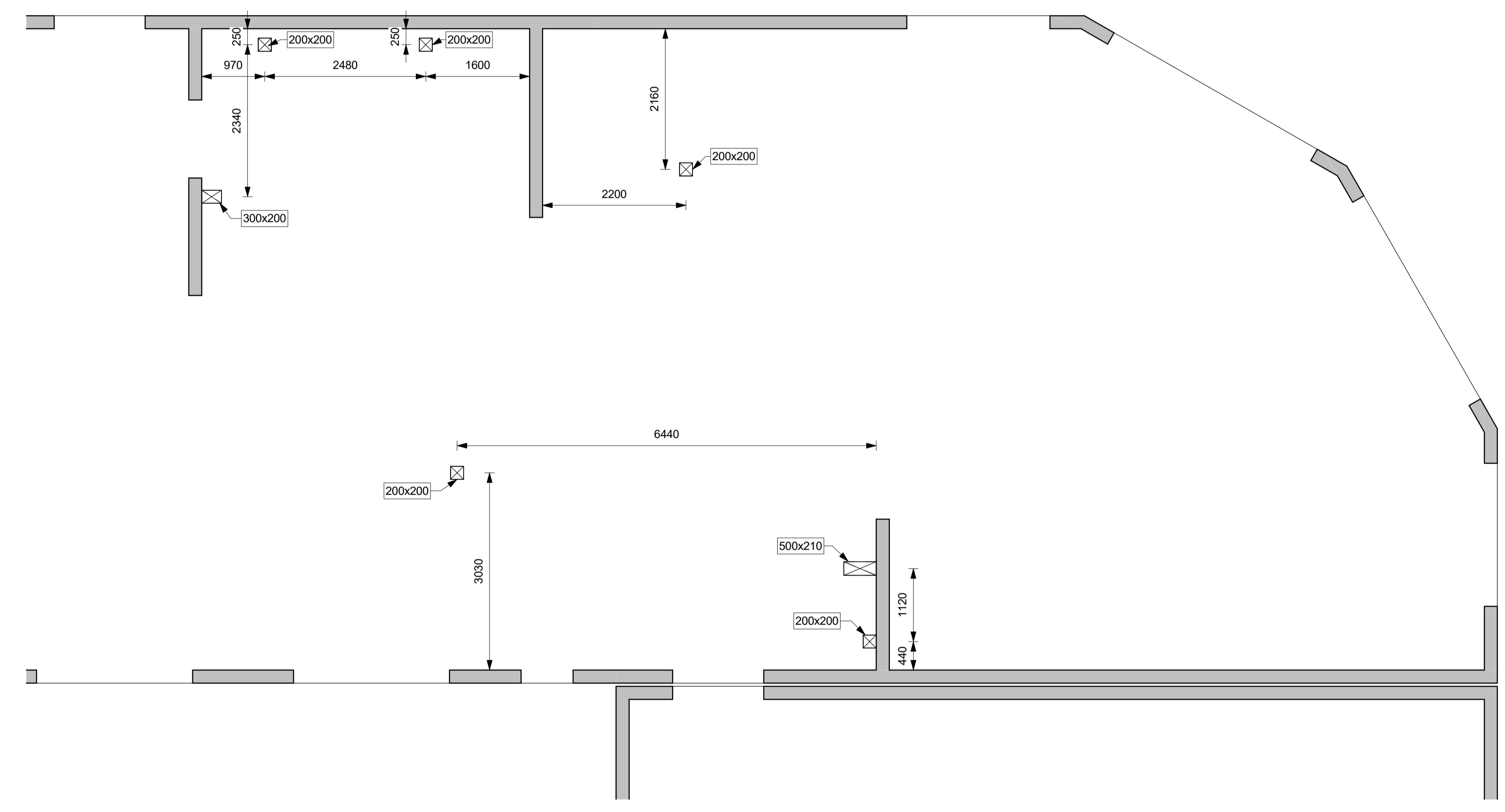
BOTNPLATA - GATAPLAN - Hluti 3 1:50
