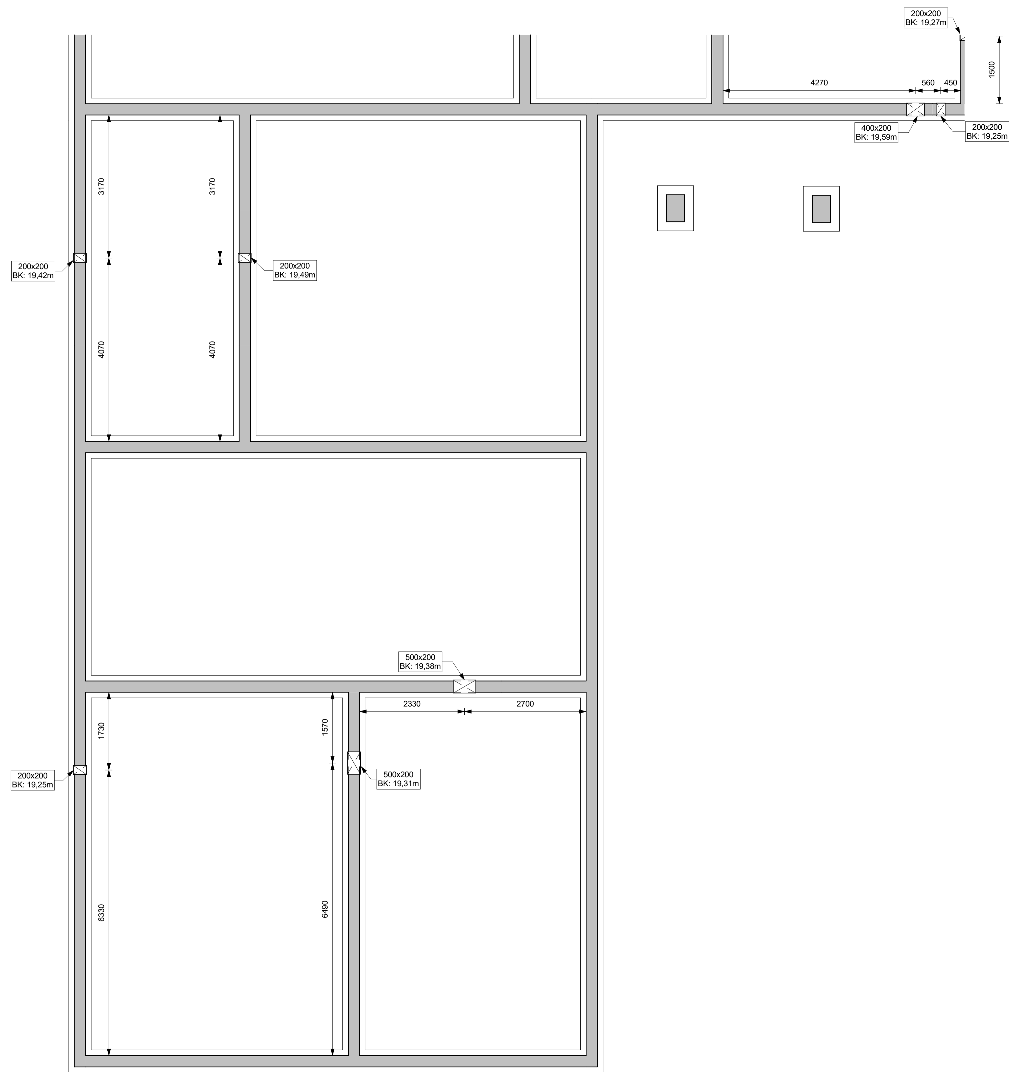
UNDIRSTÖÐUR - GATAPLAN - Hluti 1 1:50
