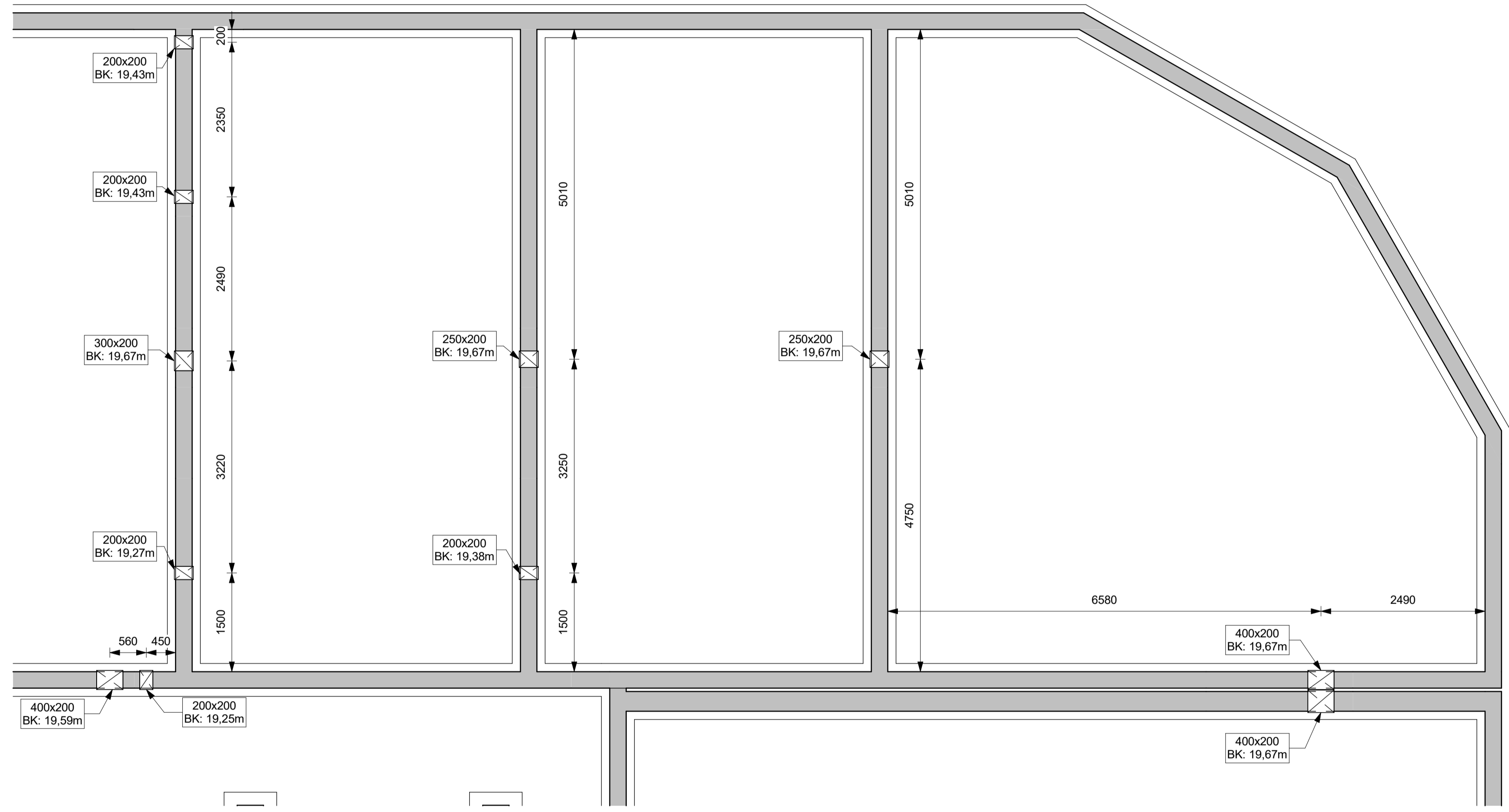
UNDIRSTÖÐUR - GATAPLAN - Hluti 3 1:50
